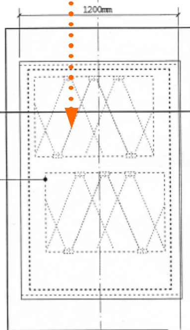
Élévation Avant type pour module A gauche
