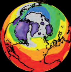
Dryas goiztiar aroa
