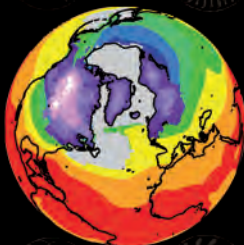
Azken glaziazio handia
